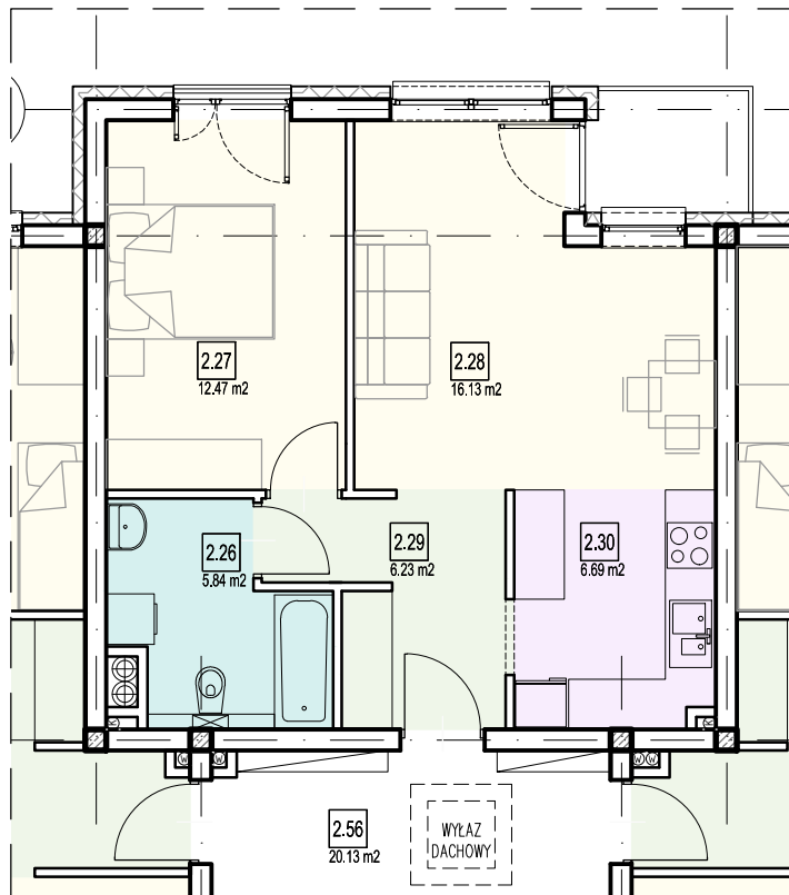
RZUT MIESZKANIA skala 1:100
