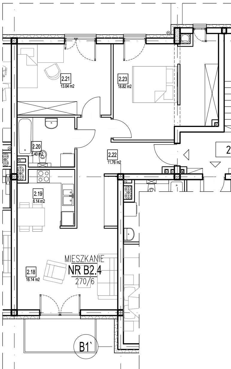
RZUT MIESZKANIA
