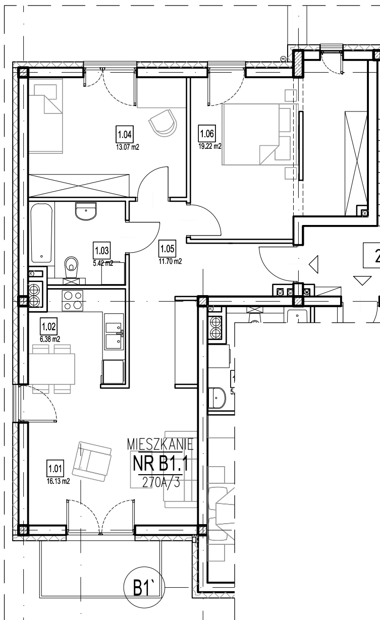
RZUT MIESZKANIA
